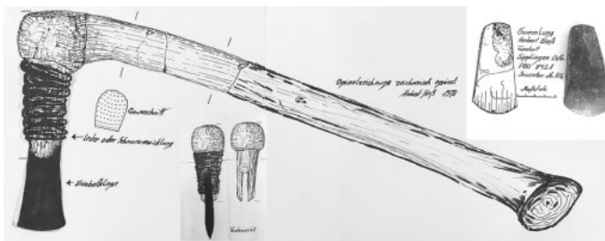
archäologische Zeichnung des Axtholms mit zeichnerischer Rekonstruktion der gesamten Axt
